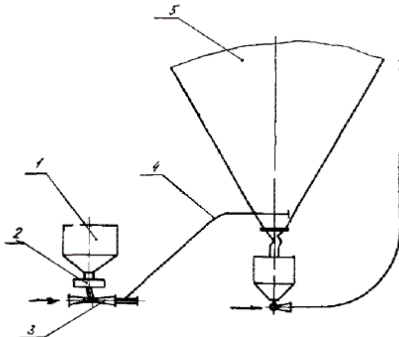
Рис. 23. Схема загрузки дроби в отдельный контур:
