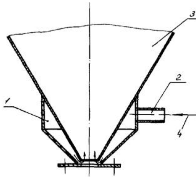
Рис. 22. Горячая рубашка:
