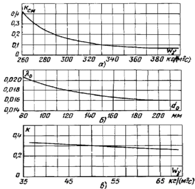
Рис. 34. Номограммы для определения коэффициентов сопротивления:
