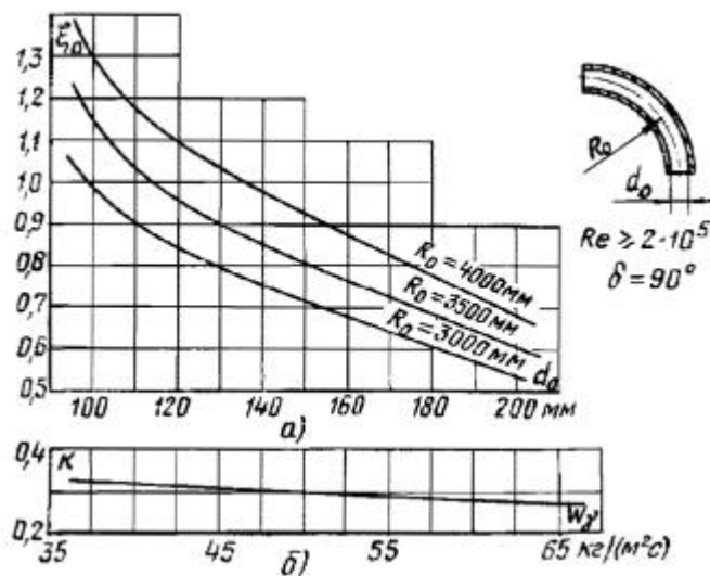
Рис. 36. Коэффициент сопротивления для колена:
