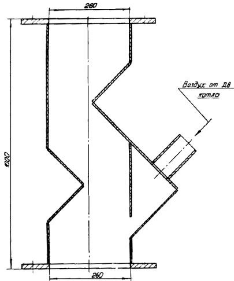
Рис. 20. Отвеиватель для котлов, работающих под наддувом
