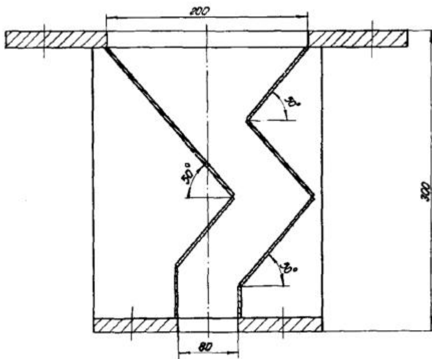
Рис. 9. Отвеиватель
