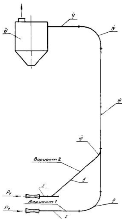
Рис. 31. Схема разбивки пневмотранспортной линии для аэродинамического расчета
