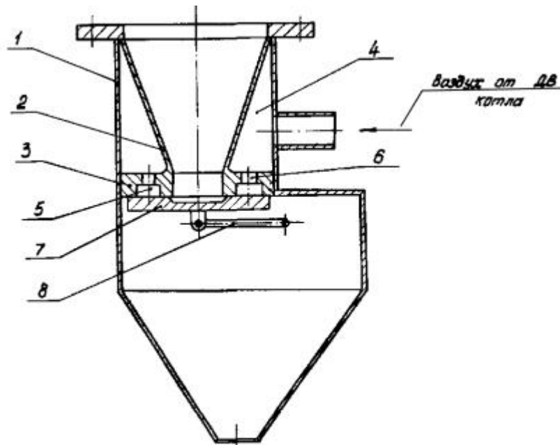
Рис. 18. Отсекатель газов:
