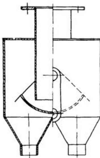
Рис. 25. Распределитель
