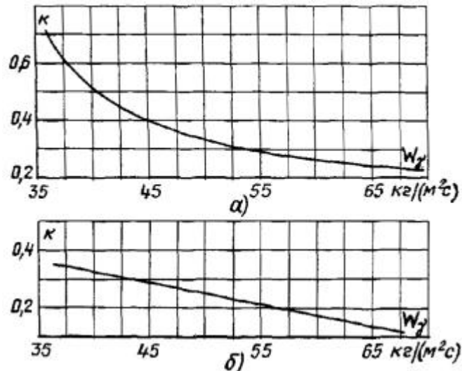
Рис. 37. Коэффициент сопротивления дроби:
