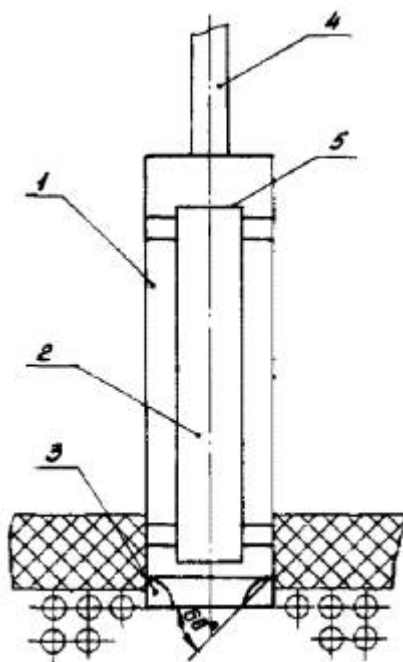
Рис. 7. Потолочный разбрасыватель дробы:
