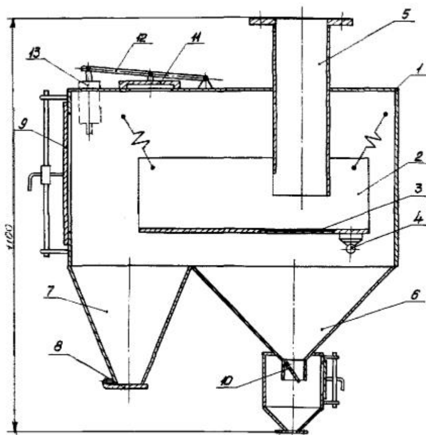
Рис. 10. Сепаратор:
