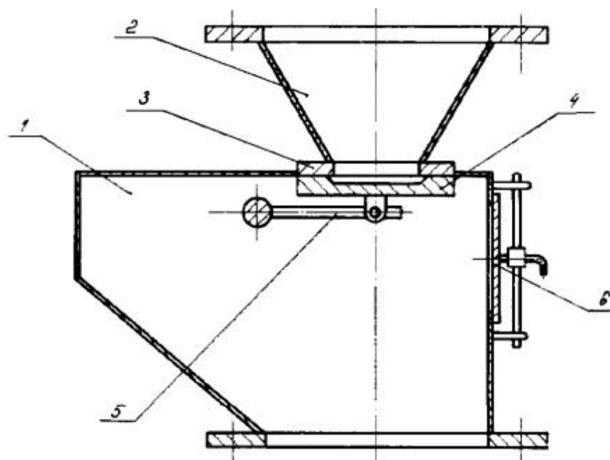
Рис. 19. Затвор:
