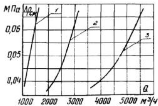
Рис. 33. Сопротивление смесителя в зависимости от расхода воздуха:
