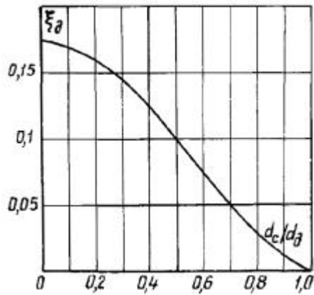
Рис. 32. Коэффициент сопротивления воздуха для диффузора с углом при вершине \alpha = 8 \square 10^\circ
