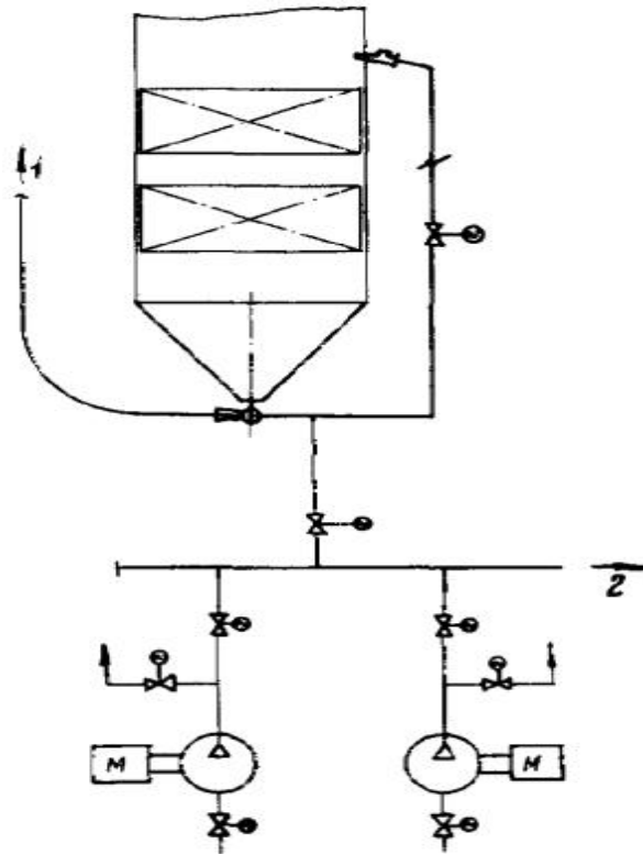
Рис. 17. Схема снабжения воздухом для пневмотранспортирования и пневмозаброса дробей:
