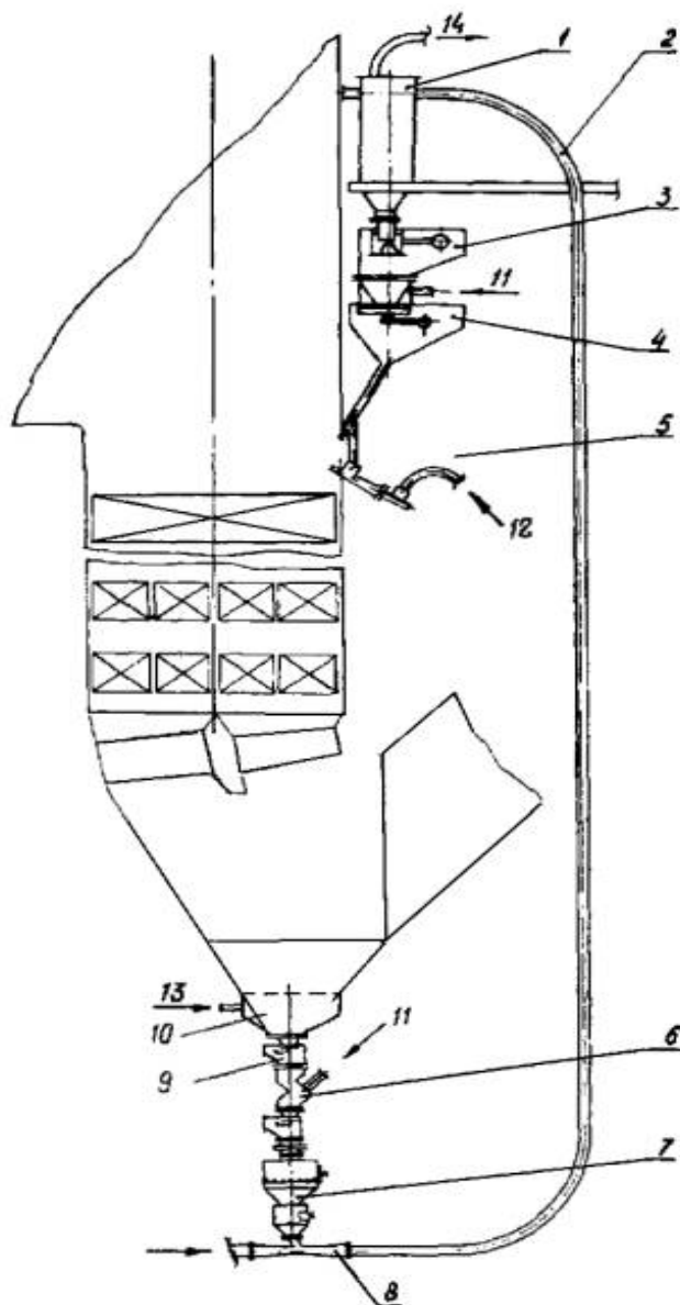
Рис. 3. Установка дробевоы очистки для котлов под наддувом:
