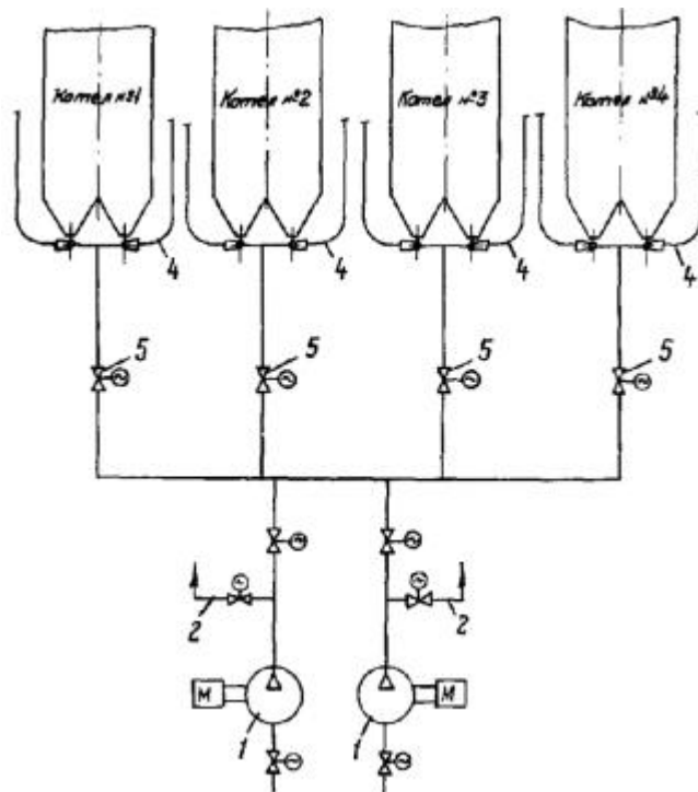
Рис. 15. Схема централизованного пневмотранспортирования дробы:
