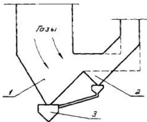
Рис. 28. Газоход за конвективной шахтой с дополнительным бункером:
