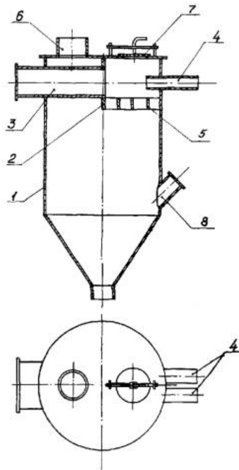
Рис. 4. Дробеуловитель:
