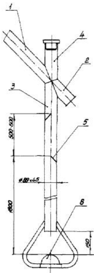
Рис. 6. Разбрасыватель дробы с полусферическим отражателем:
