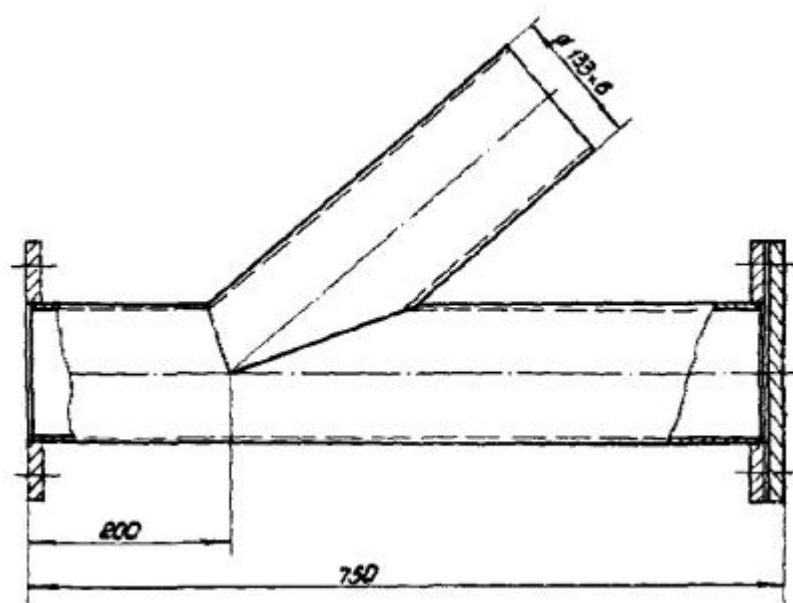
Рис. 14. Переход
