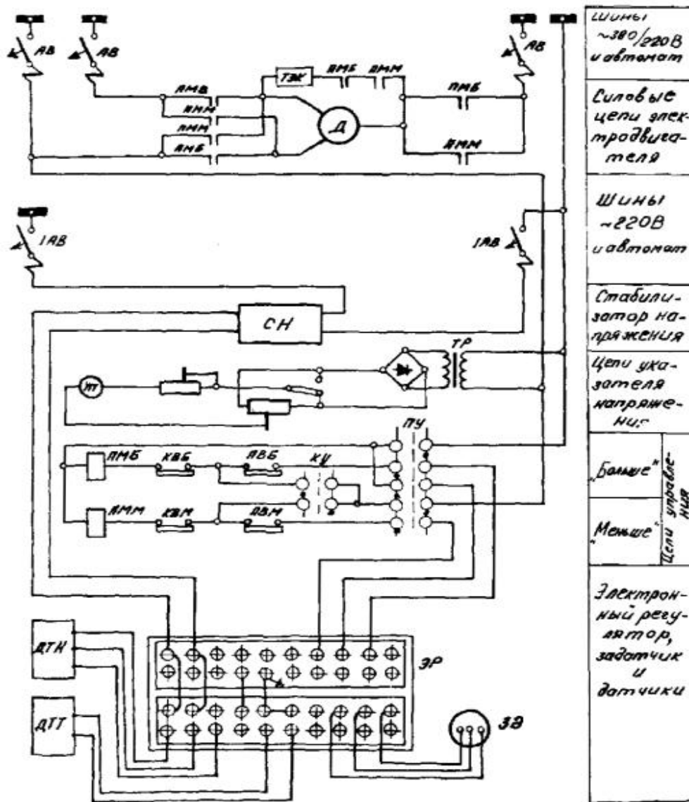
Рис. 16. Электрическая схема автоматизации противопомпажного клапана
