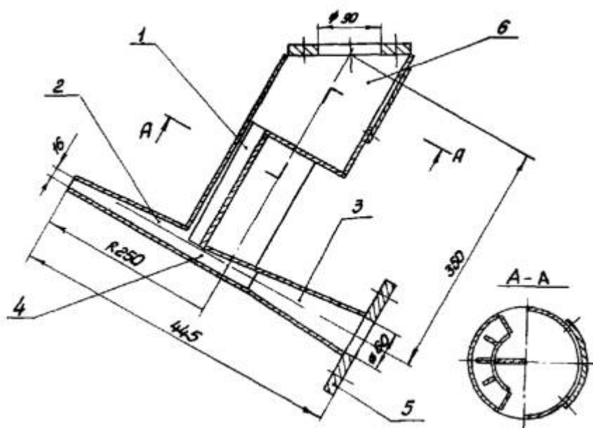
Рис. 8. Пневматический разбрасыватель дробы:
