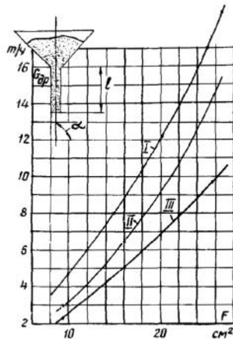
Рис. 12. Расходные характеристики патрубков загрузочных устройств:
