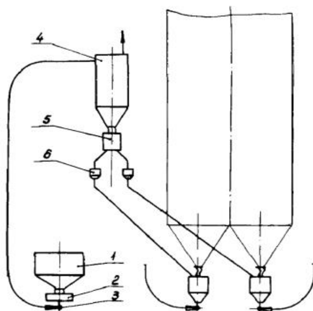
Рис. 24. Схема загрузки дроби в контуры дробеструйной установки:
