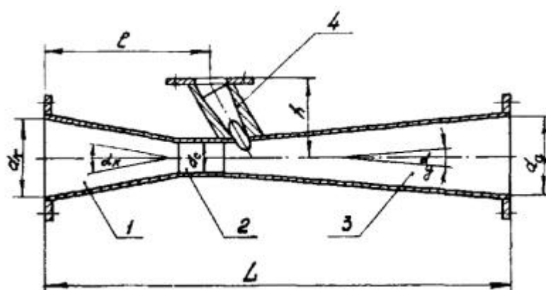
Рис. 11. Смеситель Вентури:
