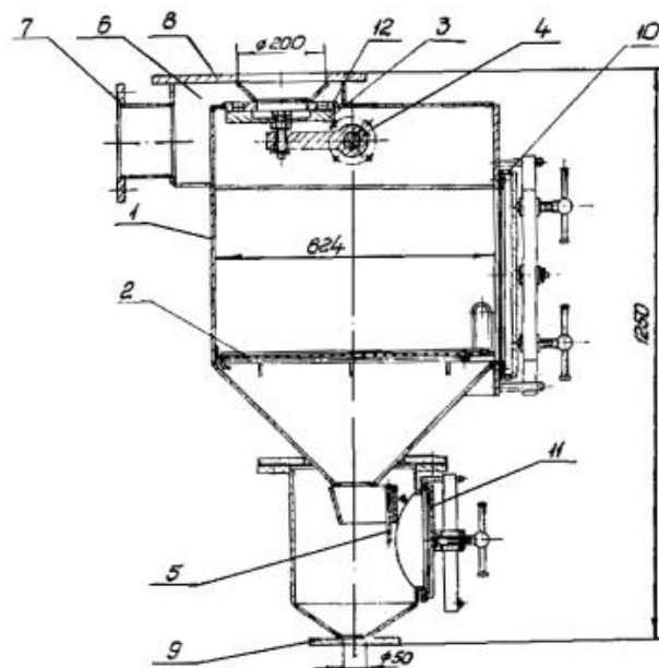
Рис. 21. Сепаратор с клапаном:
