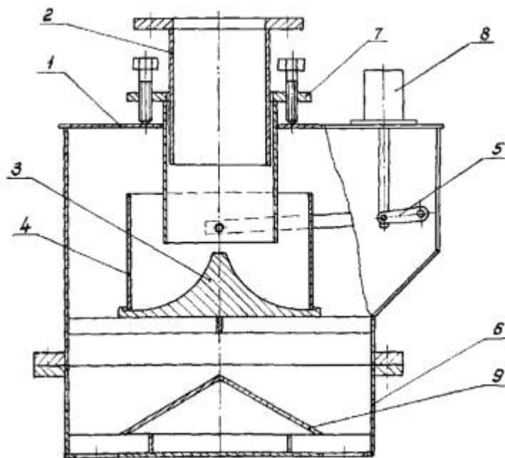
Рис. 5. Питатель дробы:
