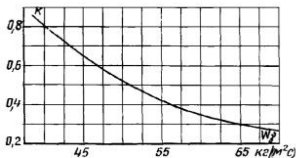
Рис. 38. Коэффициент сопротивления дроби для наклонного участка
