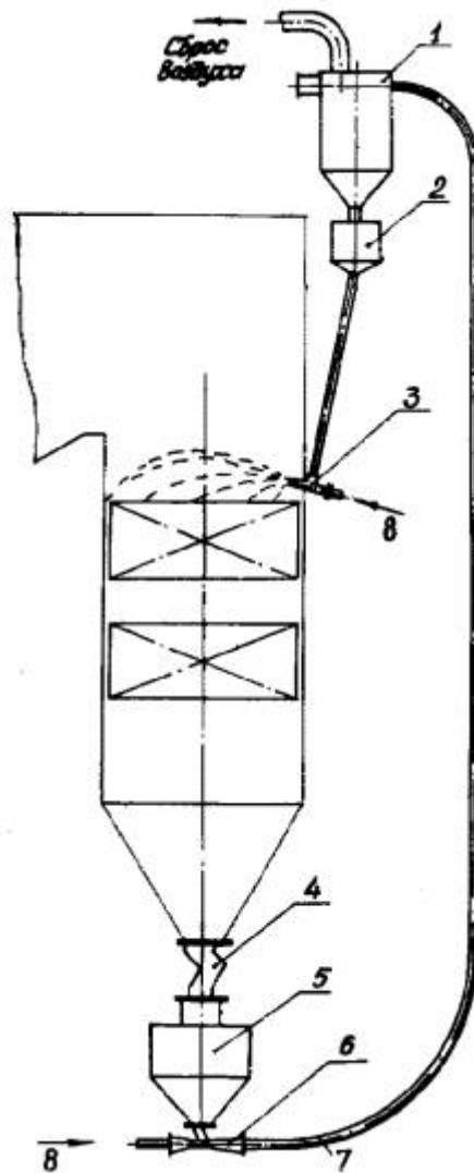
Рис. 2. Установка дробевой очистки с пневматическим разбросом:
