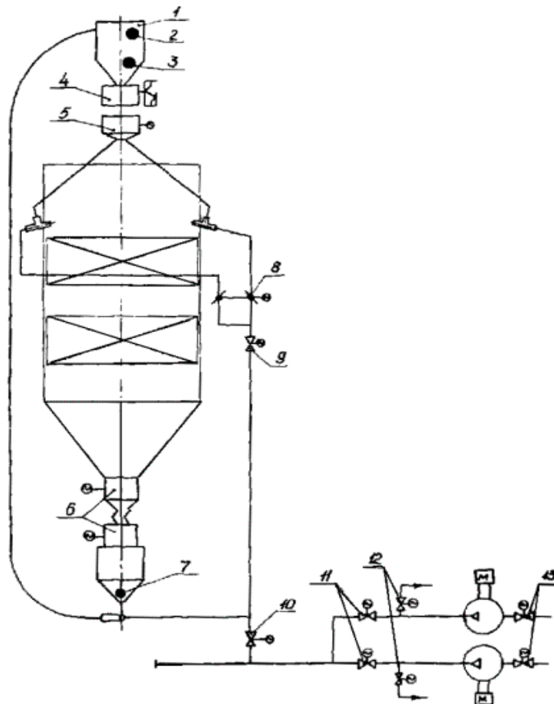
Рис. 27. Технологическая схема автоматического управления дробевой очисткой:
